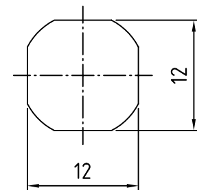
A-A部断面
